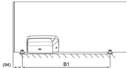
Verschillende bevestigingsmogelijkheden
