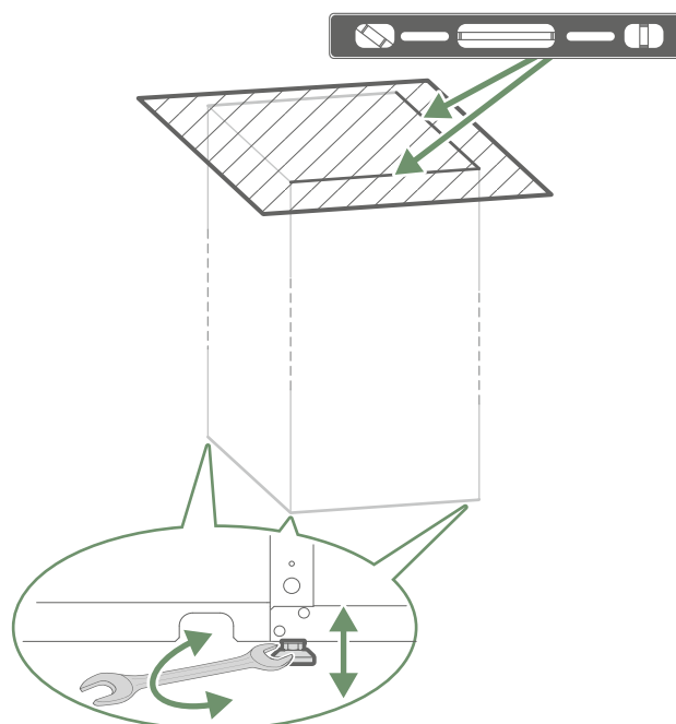
fig. 8 - Waterpas zetten
