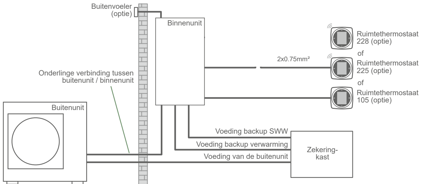
fig. 12 - Overzichtsschema van de elektrische aansluitingen voor een enkelvoudige installatie (1 verwarmingscircuit)
