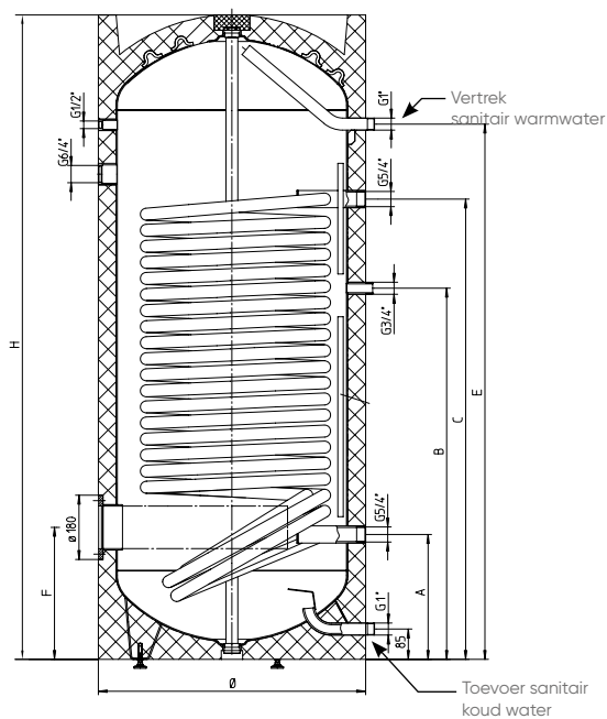
Zijaanzicht
