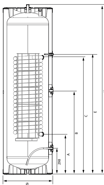
Zijaanzicht
