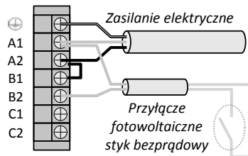
Schemat wejścia styków bezprądowych
