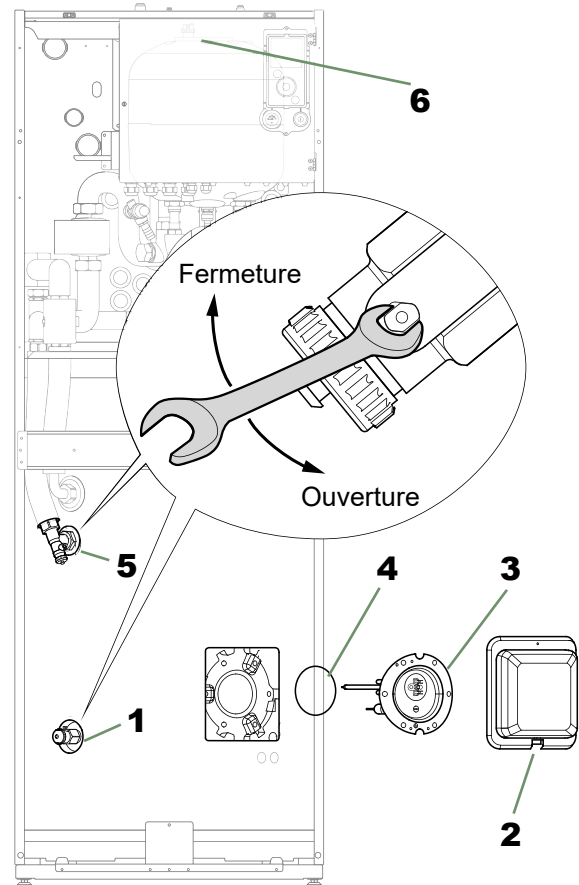
fig. 59 - Vidange du module hydraulique et/ou du ballon sanitaire
