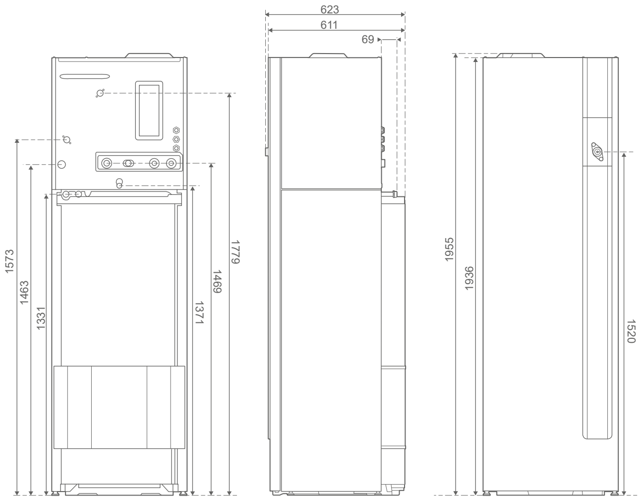
fig. 3 - Dimensions en mm
