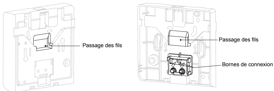
fig. 4 - Connexion des câbles
