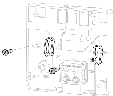
fig. 6 - Fixation au mur
