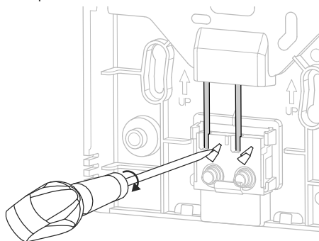
fig. 5 - Déconnexion des câbles
