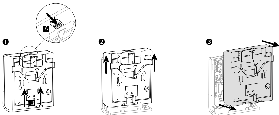
fig. 2 - Ouverture de la sonde
