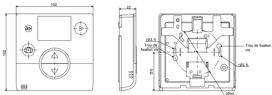
fig. 1 - Dimensions en mm
